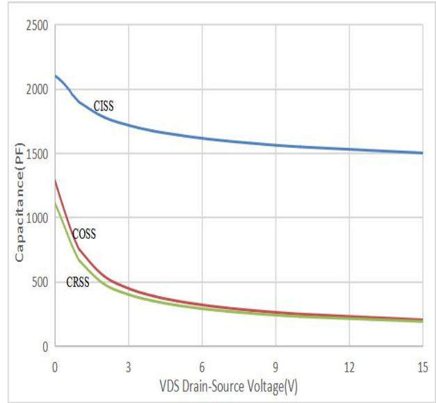
Figure 6 Capacitance Vs V DS
